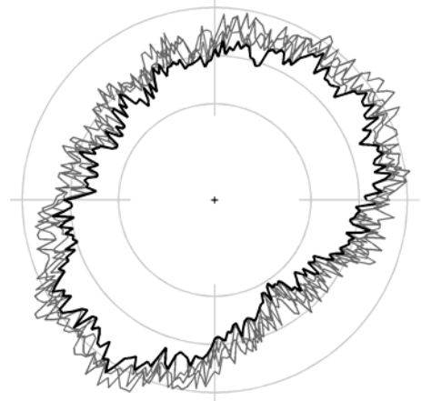
e) Inner error motion
