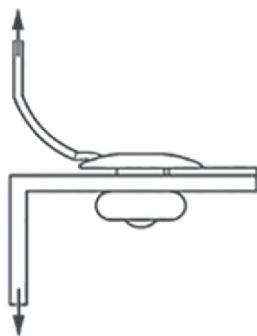
a) Sheet metal failure (Pull out)
