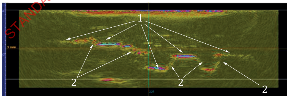
a) FMC/TFM image
