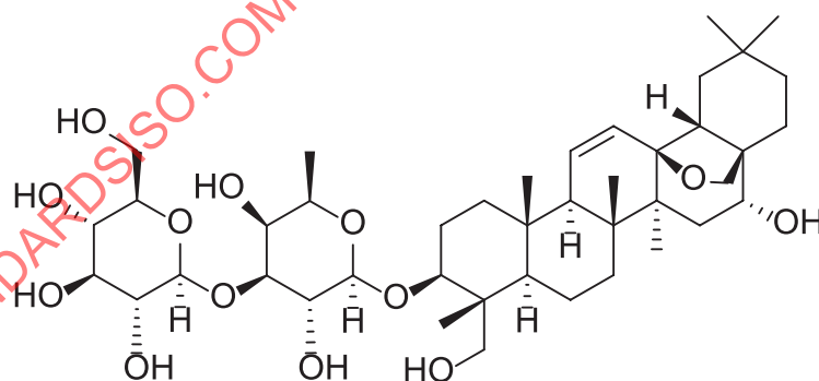
a) Saikosaponin a
