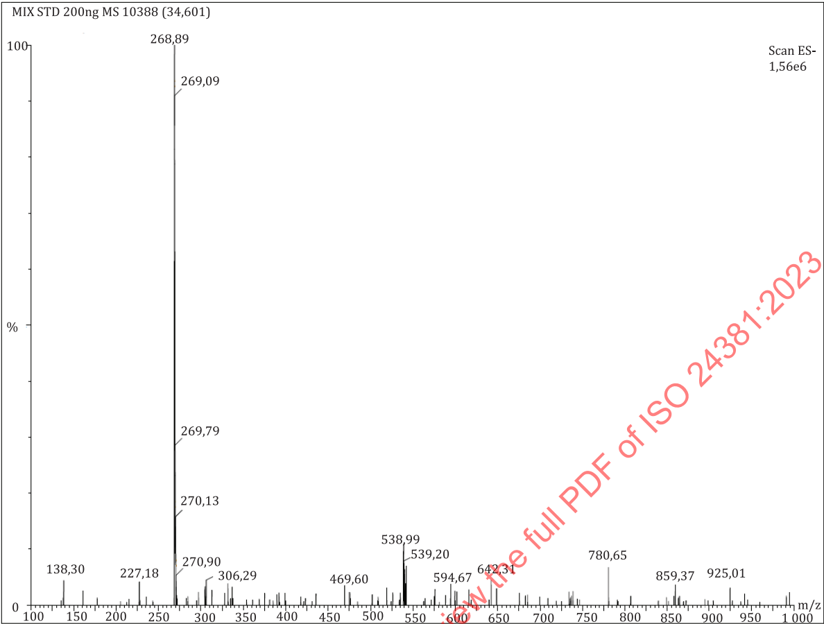
a) Apigenin
