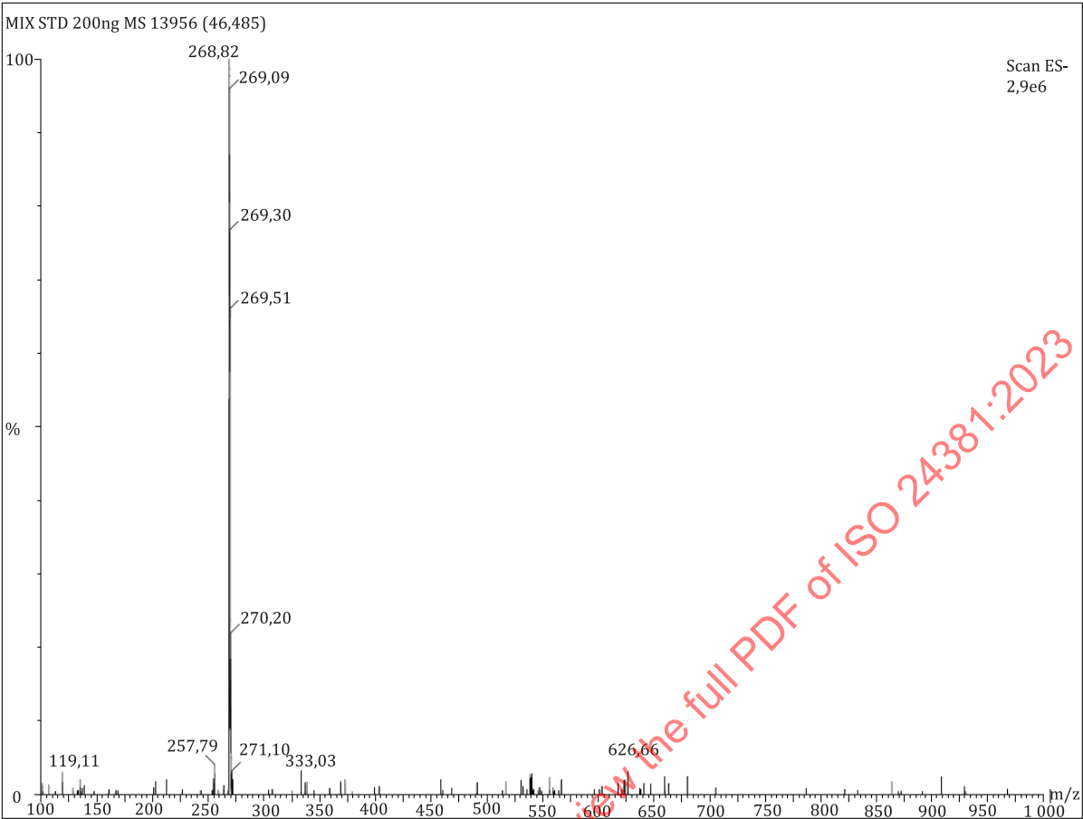
g) Galangin
