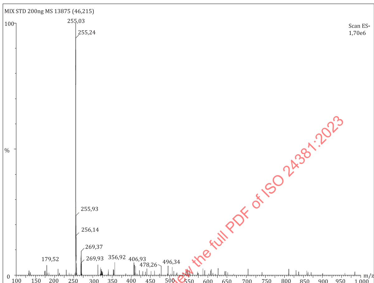
h) Pinocembrin
