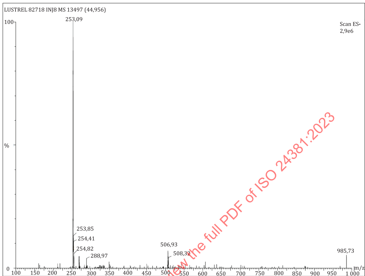
f) Chrysin
