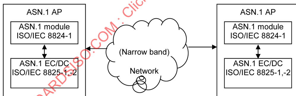
Figure F.1 — Efficient encoding using ASN.1 encoding
