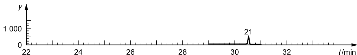
t) Ion 340
