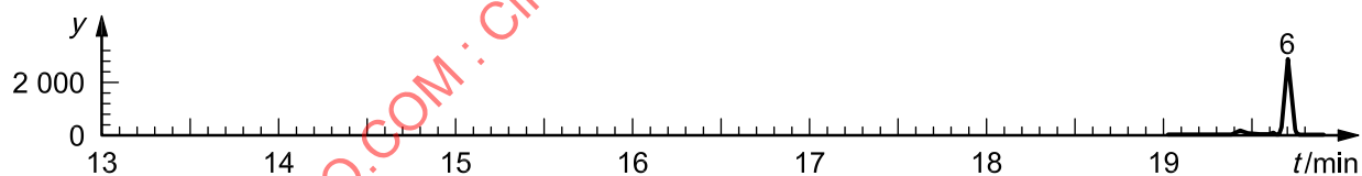
e) Ion 214
