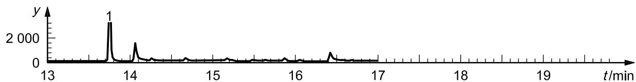
a) Ion 171
