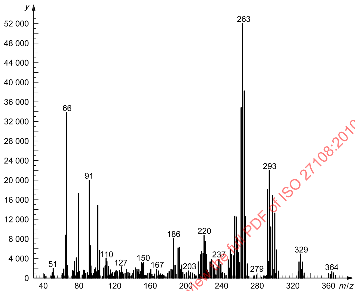
I) Aldrin
