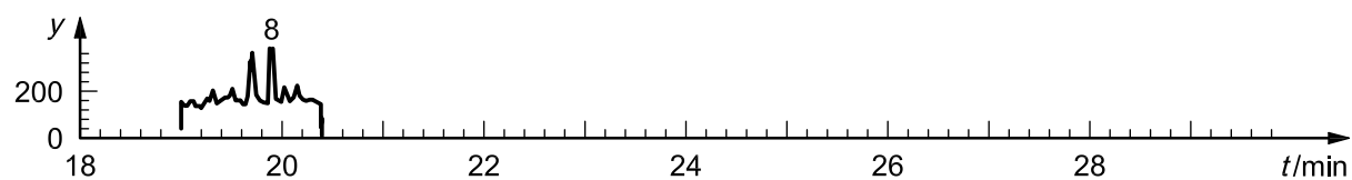
h) Ion 181
