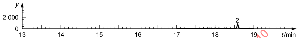
b) Ion 186
