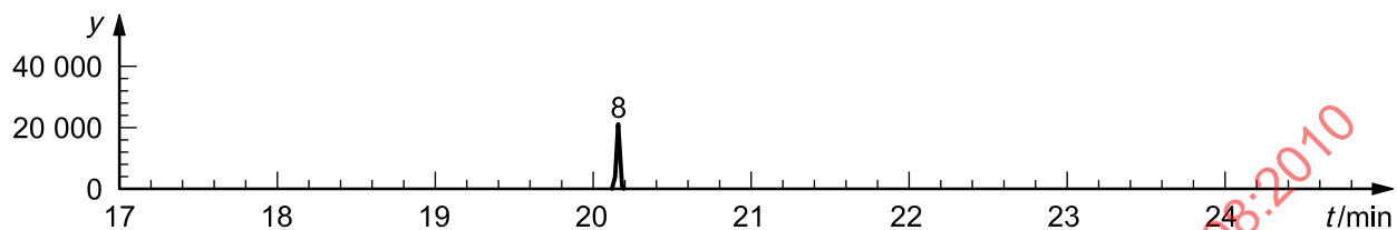
h) Ion 198
