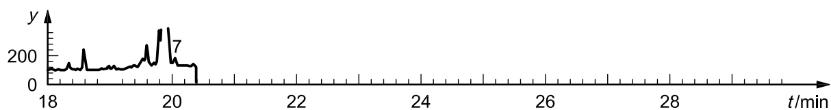
g) Ion 201
