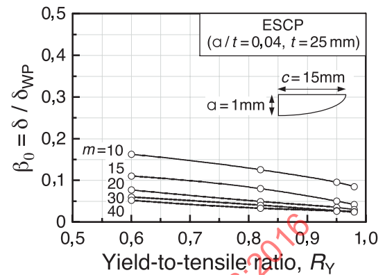
b) ESCP ( a/t = 0,24 ; t = 25 mm): \beta_0 versus R_Y
