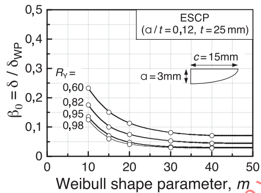
c) ESCP ( a/t = 0,12 ; t = 25 mm): \beta_0 versus m
