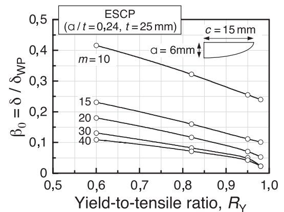
f) ESCP ( a/t = 0,24 ; t = 25 mm): \beta_0 versus R_Y
