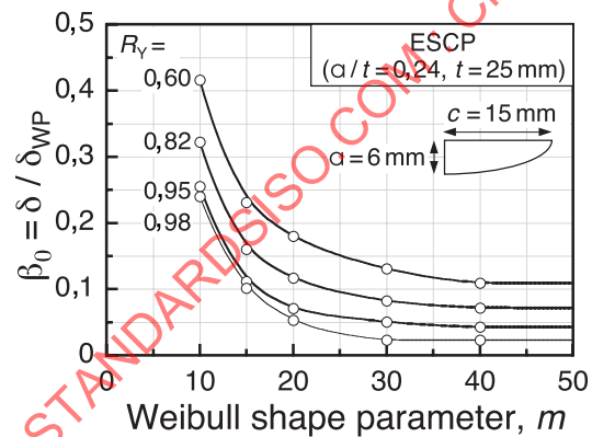
e) ESCP ( a/t = 0,24 ; t = 25 mm): \beta_0 versus m
