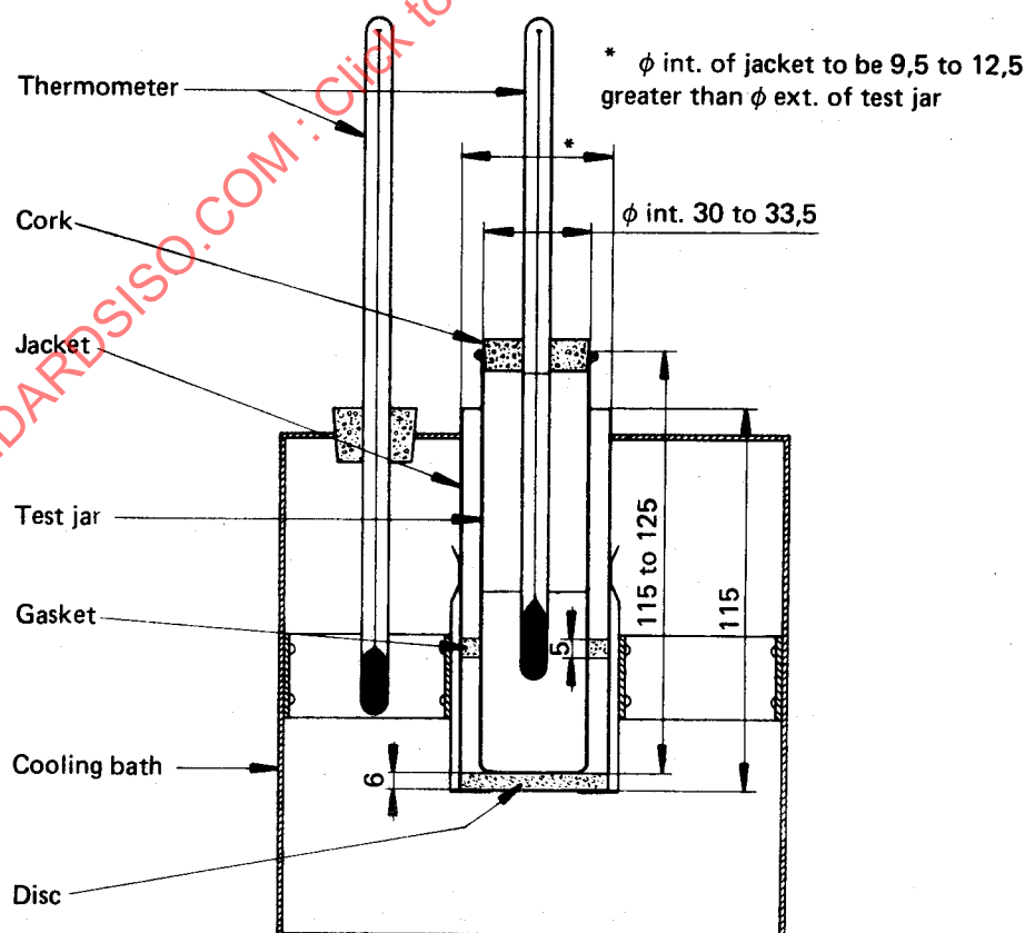
FIGURE — Apparatus for pour point test
