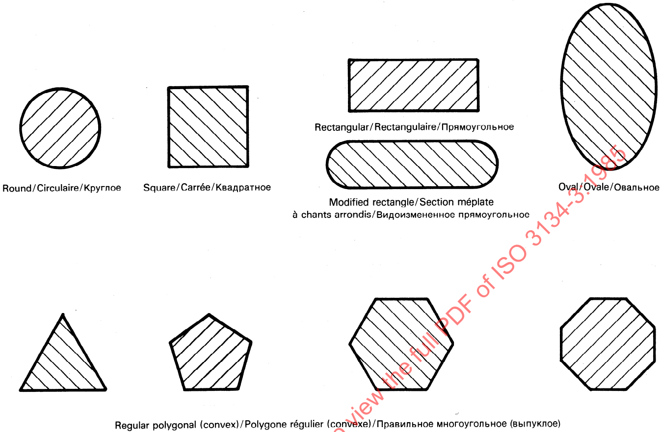
Figure 1 — Rod/bars and wire cross-sections/ Figure 1 — Sections transversales des barres et fils/ Рисунок 1 — Поперечные сечения прутков, мелких сортов и проволок
