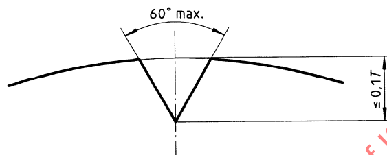
V10 notch
