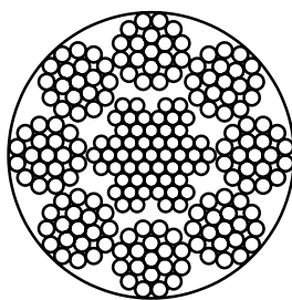
r) 8×25F-IWRC
