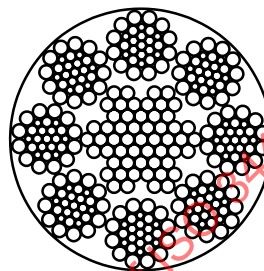
u) 8×36WS-IWRC
