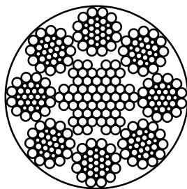
t) 8×31WS-IWRC
