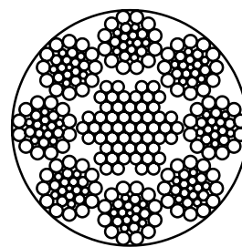
s) 8×26WS-IWRC
