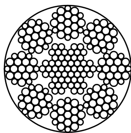
q) 8×19W-IWRC
