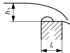
b) Short-crested weir 0,4 \leq h_1/L \leq 1,6
