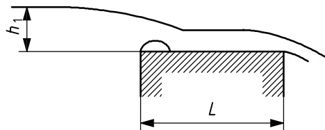
a) Broad-crested weir 0,1 \leq h_1/L \leq 0,4
