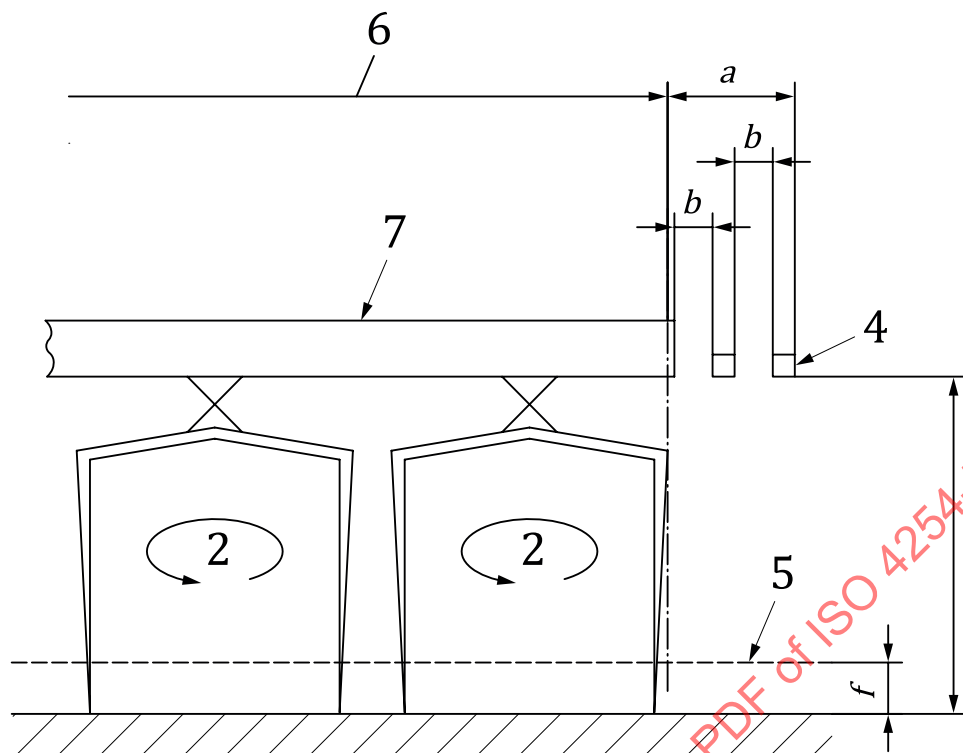
b) Side barriers (see 4.3.1)
