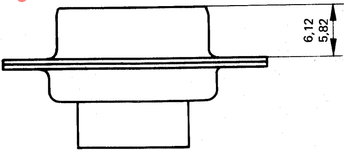
Figure 1b) — DTE 9-pin interface connector
