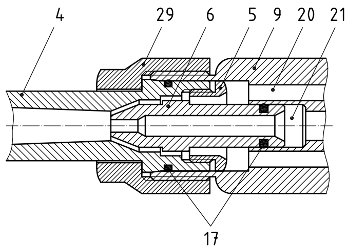
a) Injector-mixer
