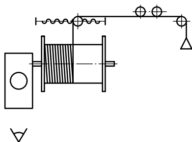
a) LVR winch
