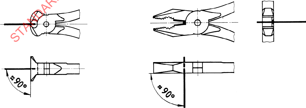
b) End cutting nipper
