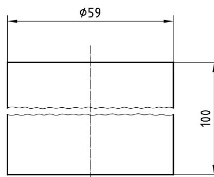
b) Plunger
