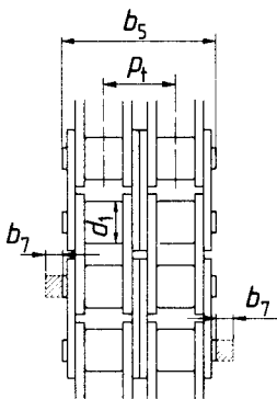
Duplex
