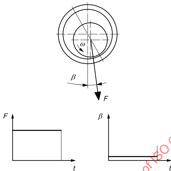
a) Static load
