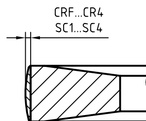
b) TB or KB rings
