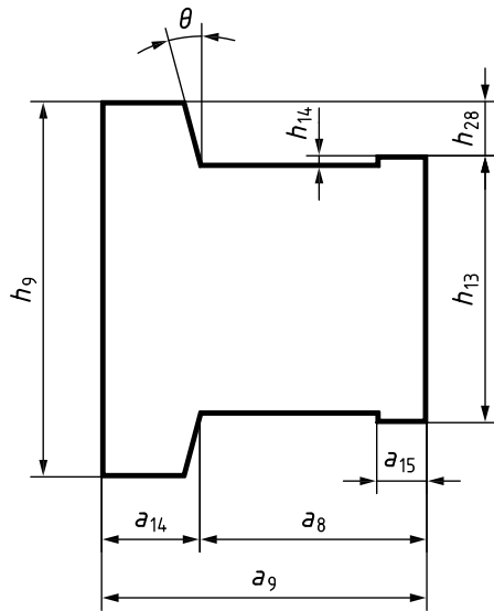
b) Expander
