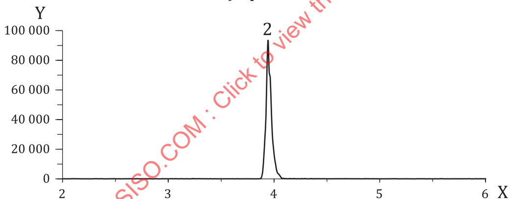
a) Fipronil
