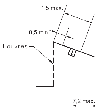
(d) Louvred ceiling or roof with louvred riser
