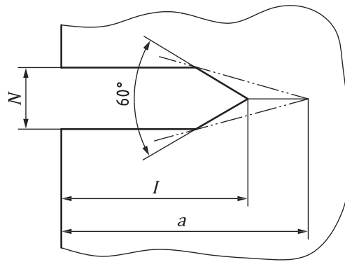
c) Bend or tensile test piece
