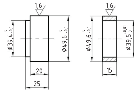
b) Piston
