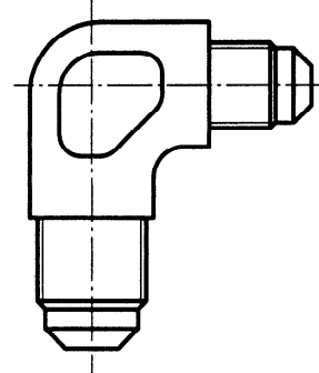
ISO 8434-2 - REE - 20 × 12
