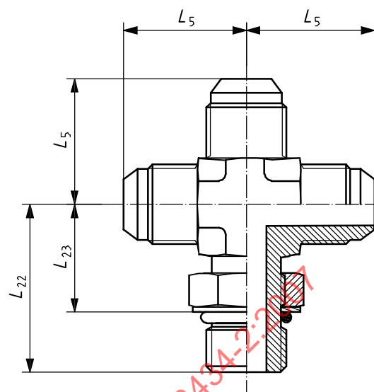
f) Adjustable stud cross (SDK)
