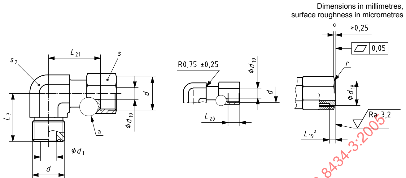
a) Swivel elbow (SWE)
