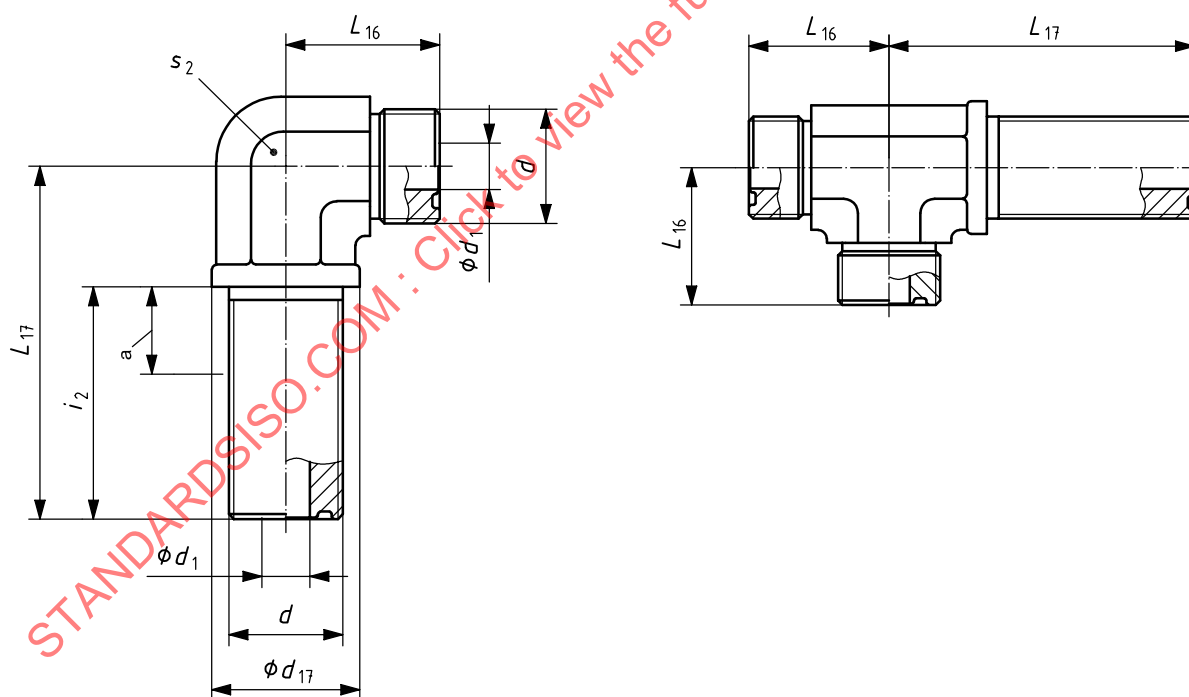
b) 90° bulkhead elbow (BHE)
