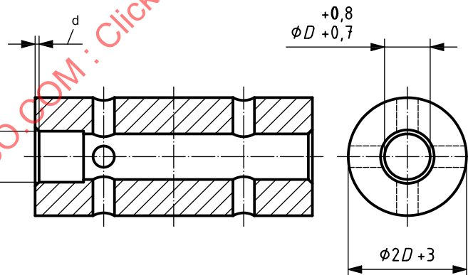
Clinch nuts
