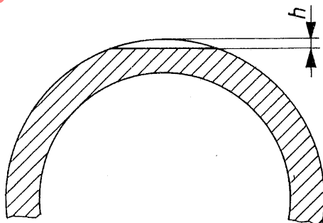
b) Chord notch
