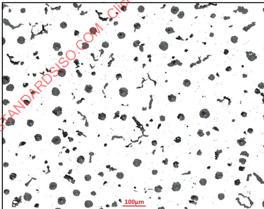
g) Nodularity 65 %
