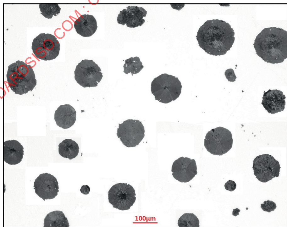
a) Maximum Féret diameter \geq 10 \mu\text{m} : 25 particles/ \text{mm}^2 ; Maximum Féret diameter \geq 5 \mu\text{m} : 31 particles/ \text{mm}^2
