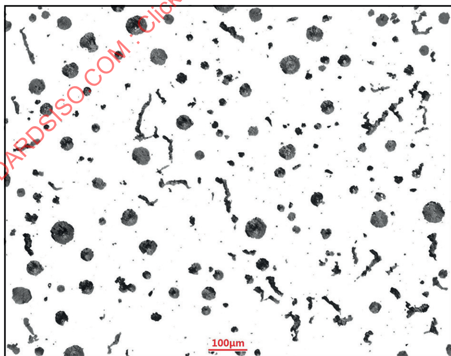
h) Nodularity 60 %
