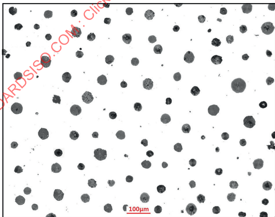
c) Maximum Féret diameter \geq 10 \mu\text{m} : 100 particles/ \text{mm}^2 ; Maximum Féret diameter \geq 5 \mu\text{m} : 116 particles/ \text{mm}^2
