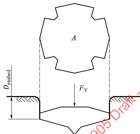
b) Actual spudcan — Fully embedded
