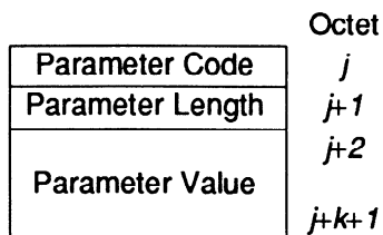
Figure 3 — Encoding of QOS Parameters
