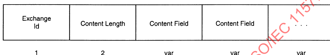
Figure C.1 – SA Contents
