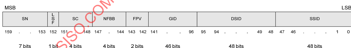
Fig. 36 - Frame Header Format
