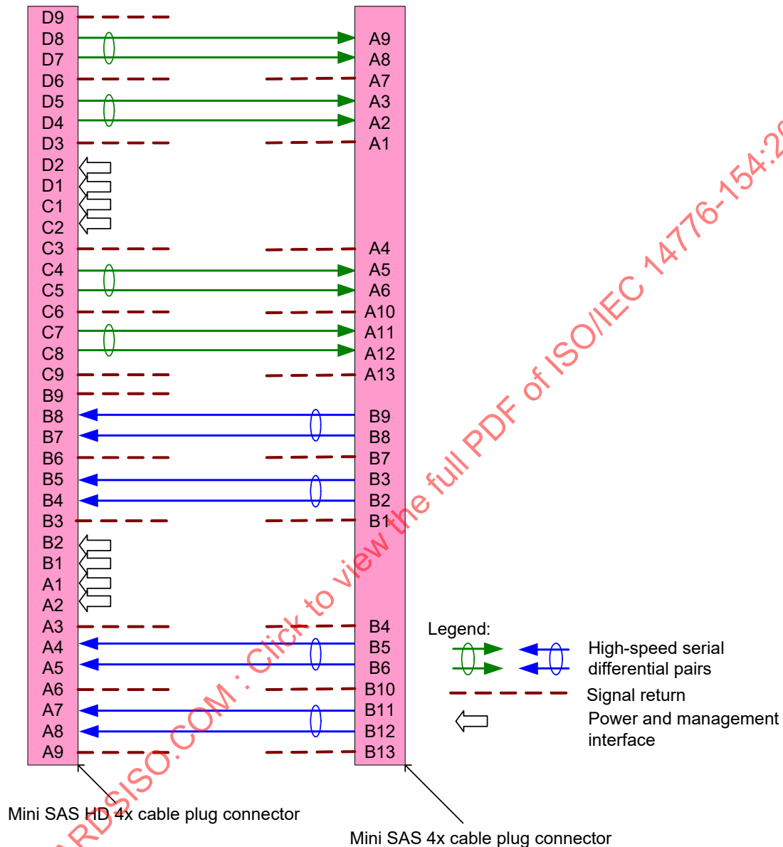
Figure 95 – SAS external cable assembly - Mini SAS HD 4x to Mini SAS 4x
