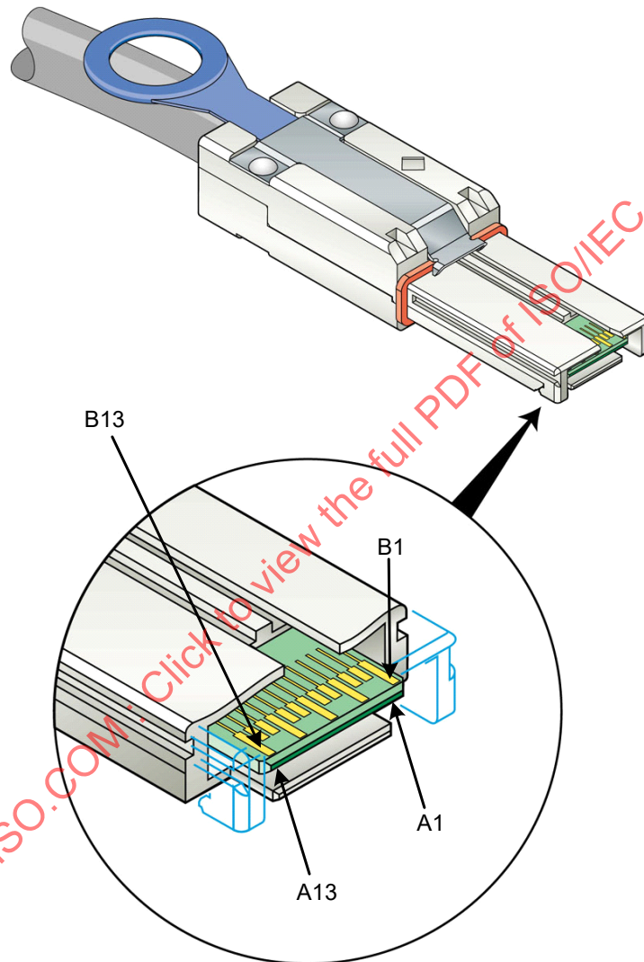
Figure 42 – Mini SAS 4x cable plug connector
