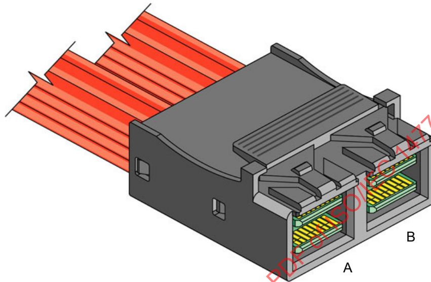
Figure 38 – Mini SAS HD 8i cable plug connector
