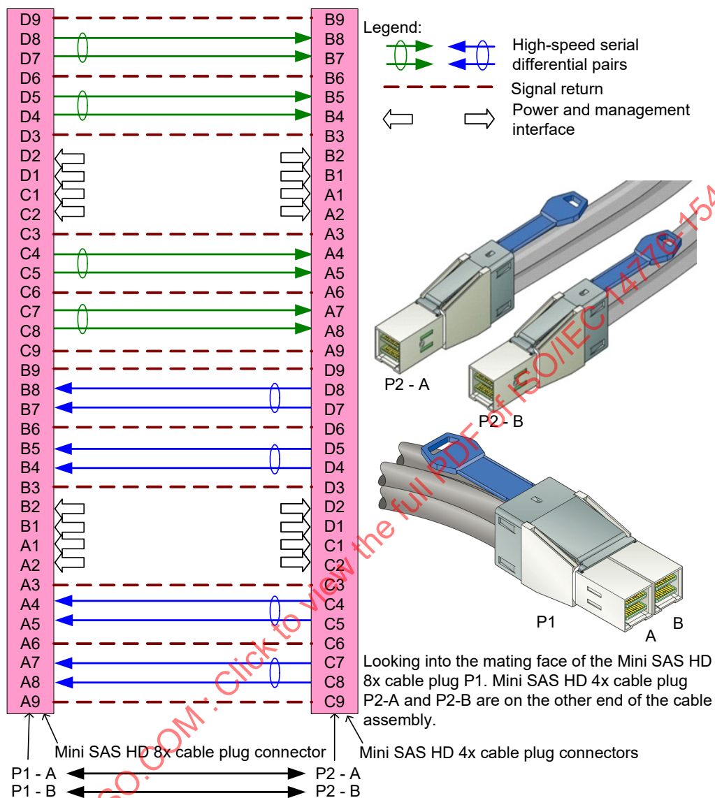
Figure 93 – SAS external cable assembly - Mini SAS HD 8x to Mini SAS HD 4x
