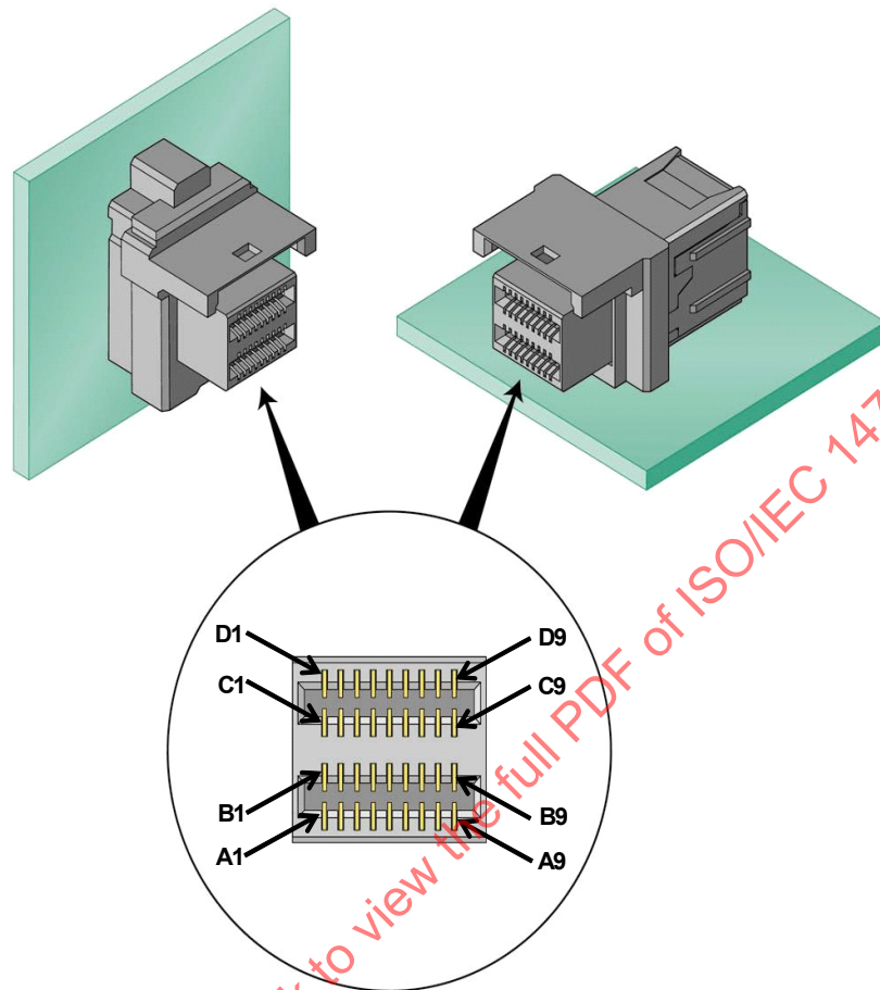
Figure 39 – Mini SAS HD 4i receptacle connector
