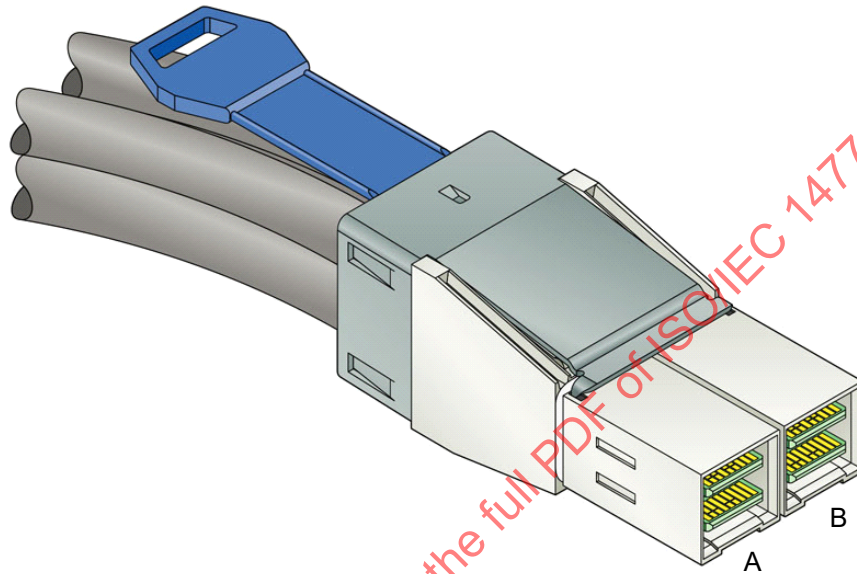
Figure 63 – Mini SAS HD 8x cable plug connector
