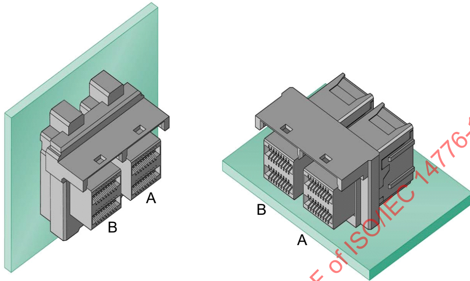
Figure 40 – Mini SAS HD 8i receptacle connector
