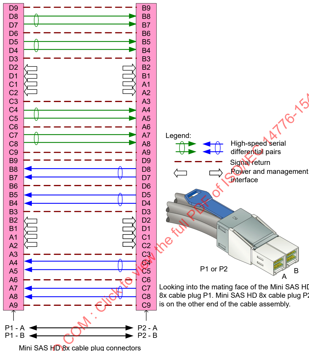
Figure 91 – SAS external cable assembly - Mini SAS HD 8x
