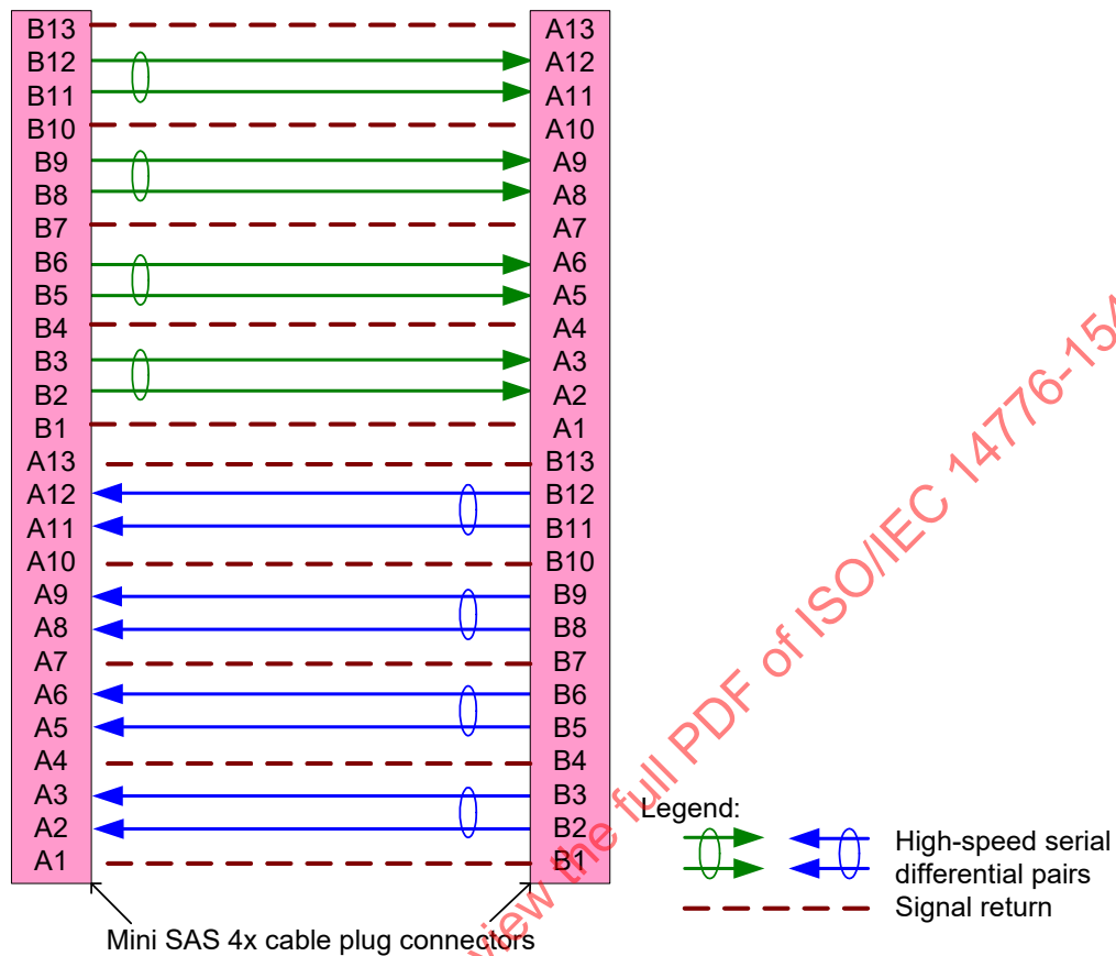
Figure 86 – Mini SAS 4x external cable assembly
