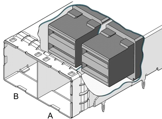
Figure 65 – Mini SAS HD 8x receptacle connector
