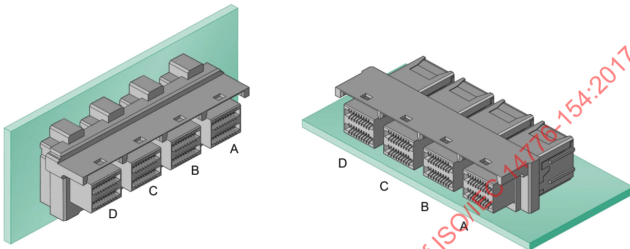
Figure 41 – Mini SAS HD 16i receptacle connector
