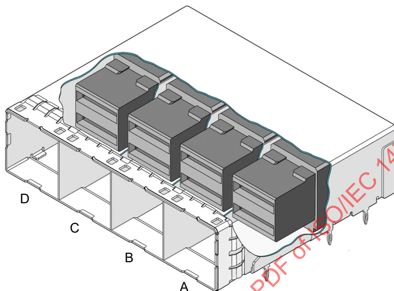
Figure 66 – Mini SAS HD 16x receptacle connector
