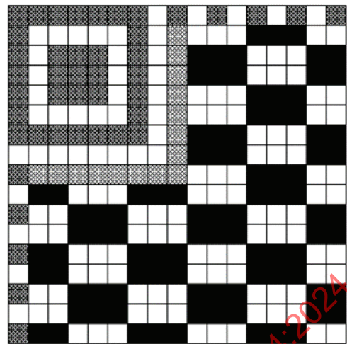
b) Mask pattern 01
