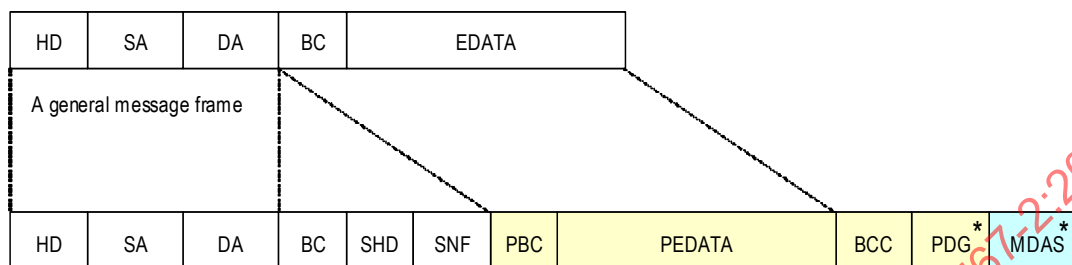
A secure message frame
