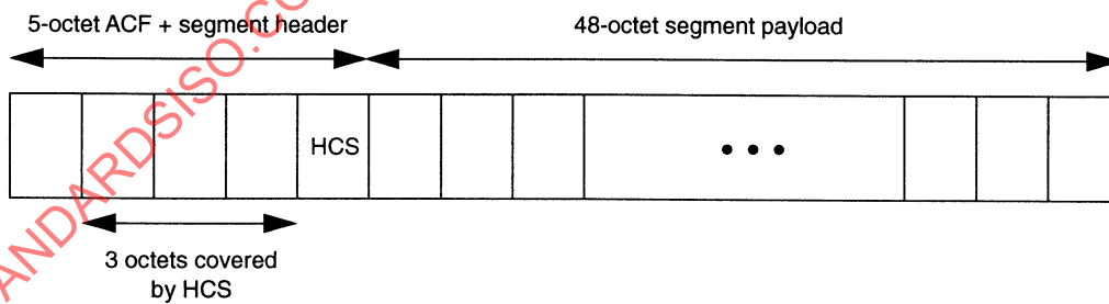
Figure 17-2—DQDB slot format
