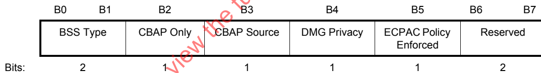
Figure 8-80c—DMG Parameters
