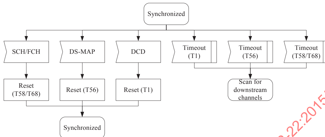
Figure 49e—Maintaining DS parameters
