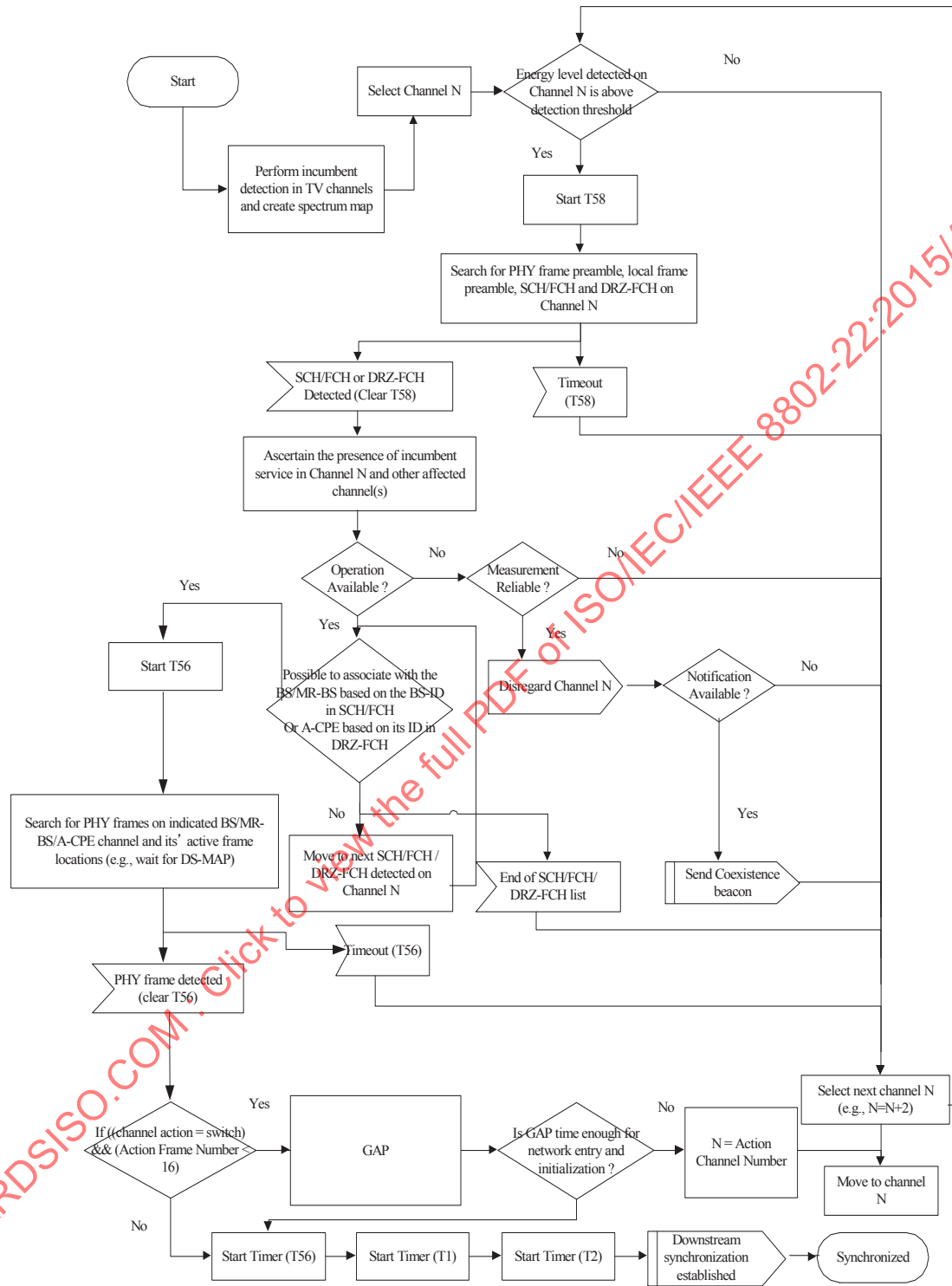
Figure 49d—Obtaining DS parameters
