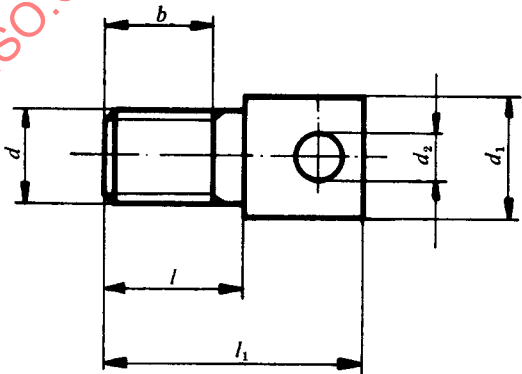
FIG. 7 — Driving bolt FIG. 7 — Vis d'entraînement Фиг. 7 — Приводной палец
