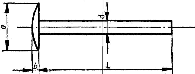
RIVET
