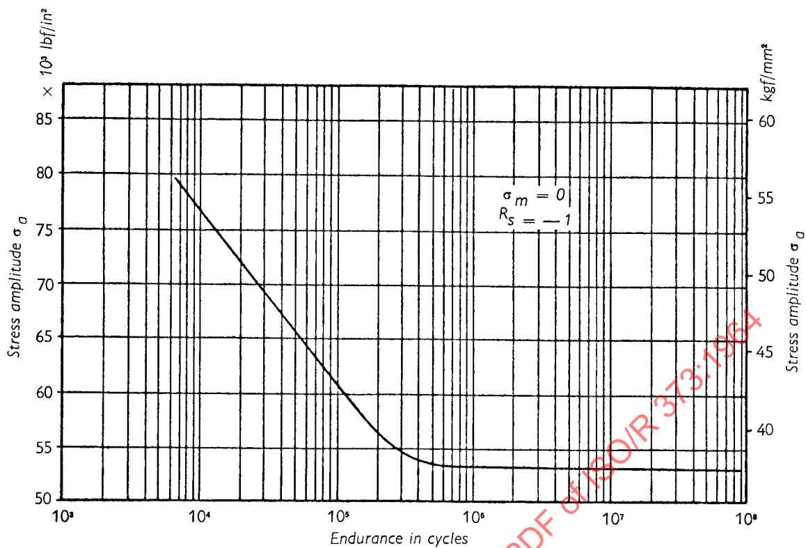
Fig. 4. — S/N curve (linear stress scale)
