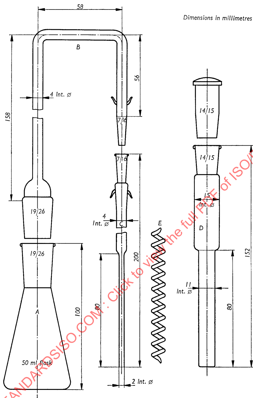
FIG. 2. — Evolution apparatus
