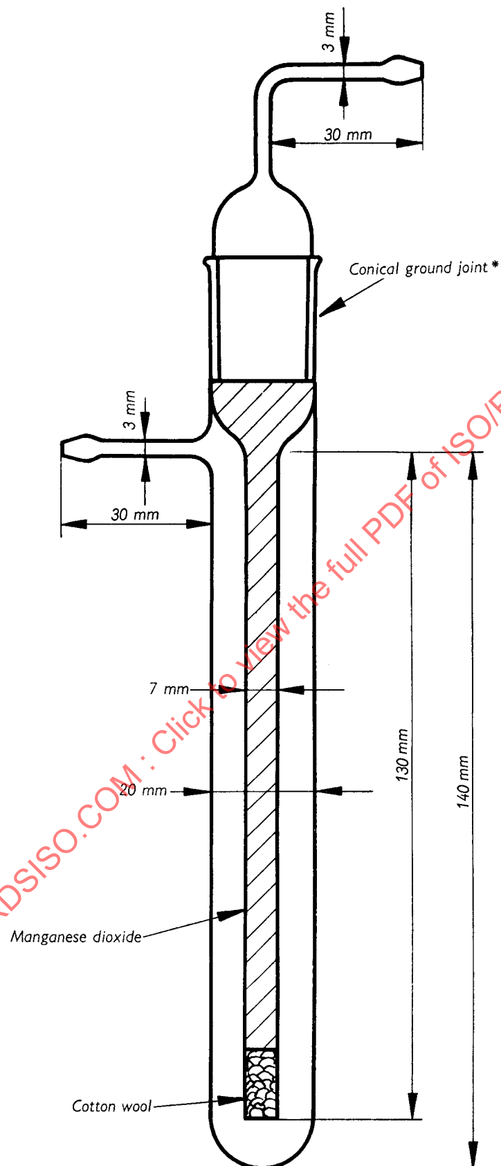
FIG. 1. — Guard-tube
