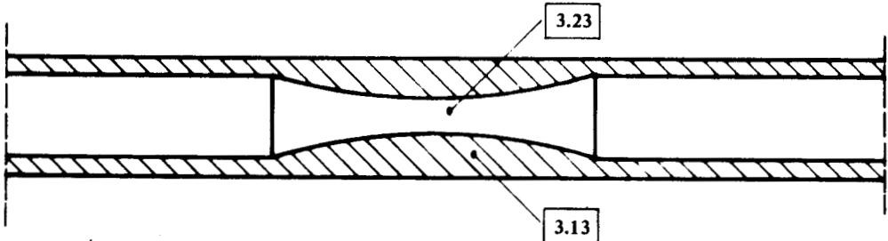
FIG. 24 – Venturi flume
